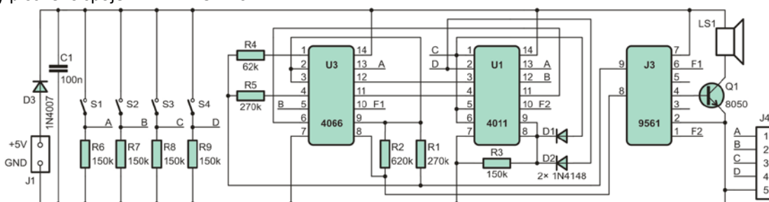
Obr. 2 schéma zapojení
